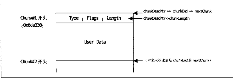
图 4-6 Sctp DATA chunk 格式
