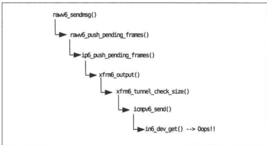
图 5-1 Oops 发生之前的调用流程
