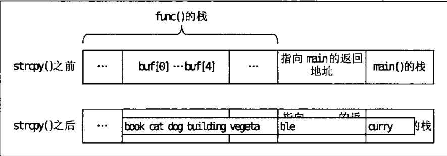
图 4-4 func()的栈
