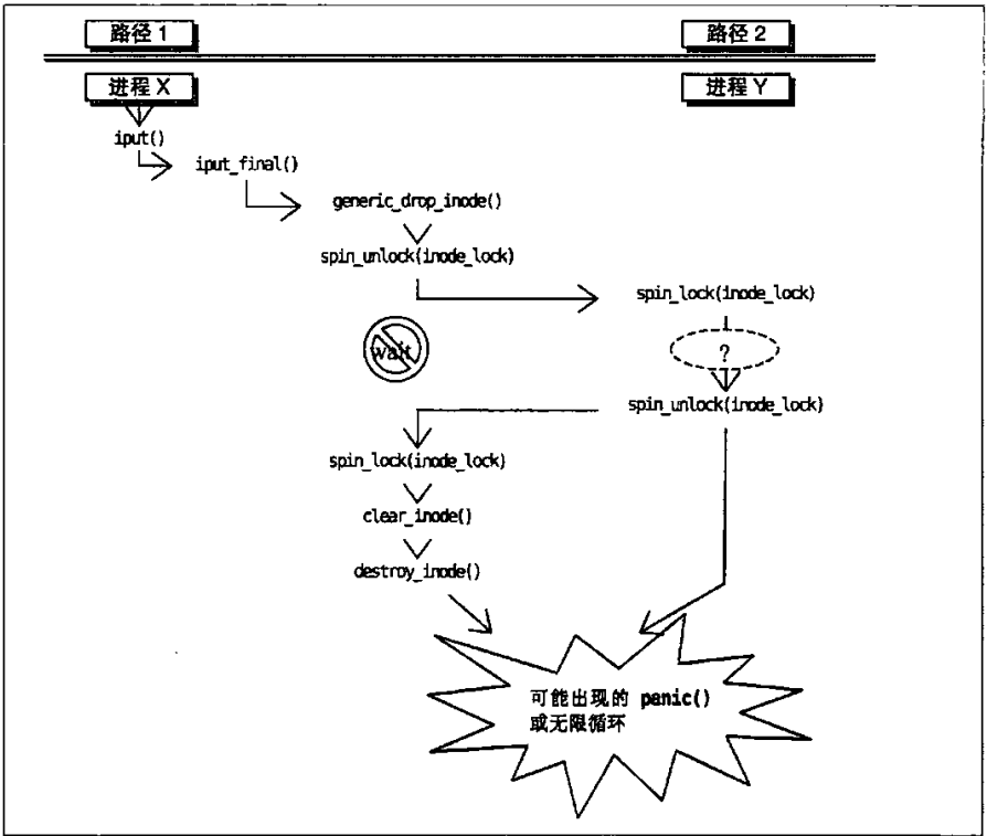
图 5-5 互斥的原理
